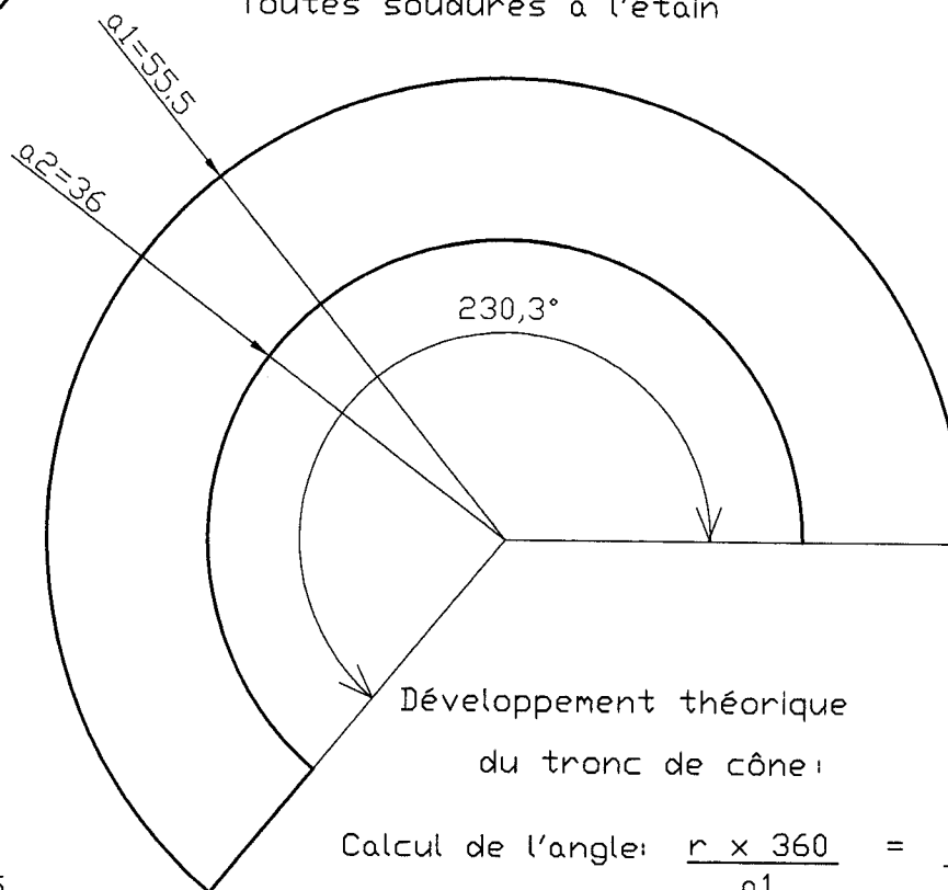
COUVERCLE
